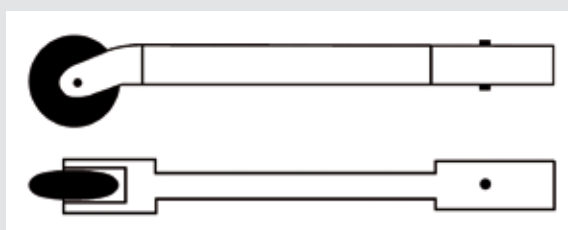
Kontaktarm 6/12 x 610 mm Bestell-Nr. 301024
