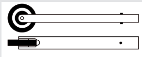
Kontaktarm 6/12 x 610 mm Bestell-Nr. 301014
