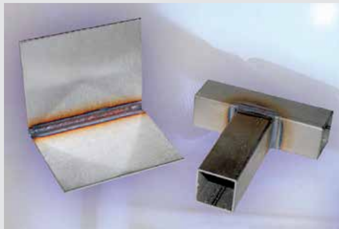
Schweißnähte vor und nach der Bearbeitung mit dem EW-Kombi Reinigungssystem
