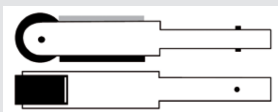
Kontaktarm 19 x 610 mm Bestell-Nr. 301030
