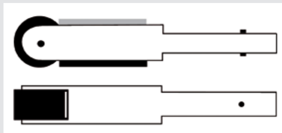
Kontaktarm 6/12 x 457 mm Bestell-Nr. 300785
